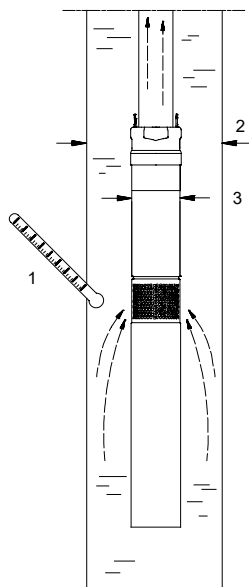
Pompă SQ/SQE într-un puț forat
